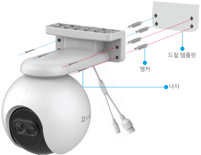
그림 2 벽 장착
