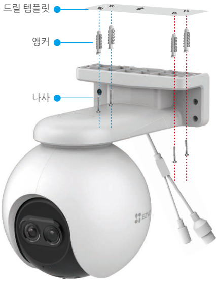
그림 1 천장 장착
